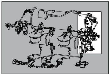
Detalle A
