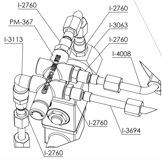
Detalle A
