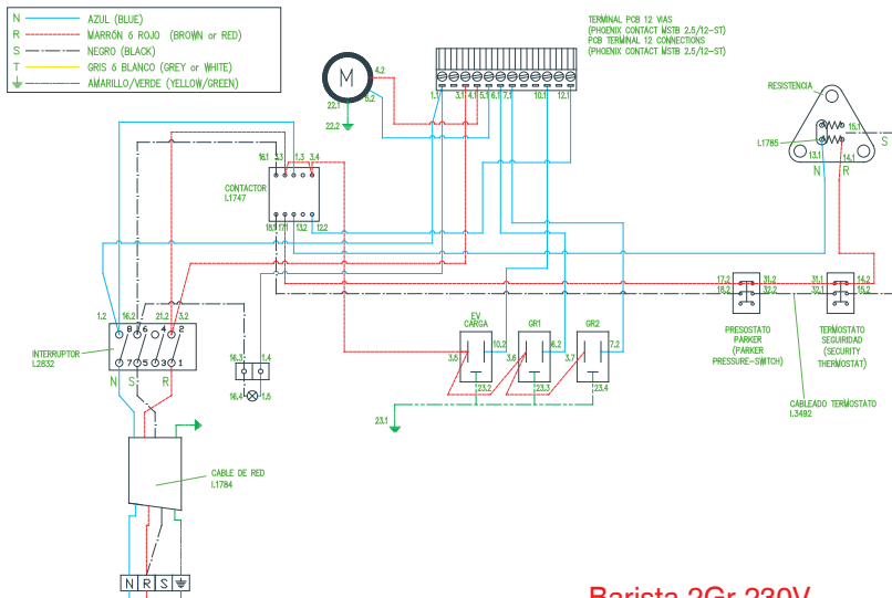
Barista 2Gr 230V
