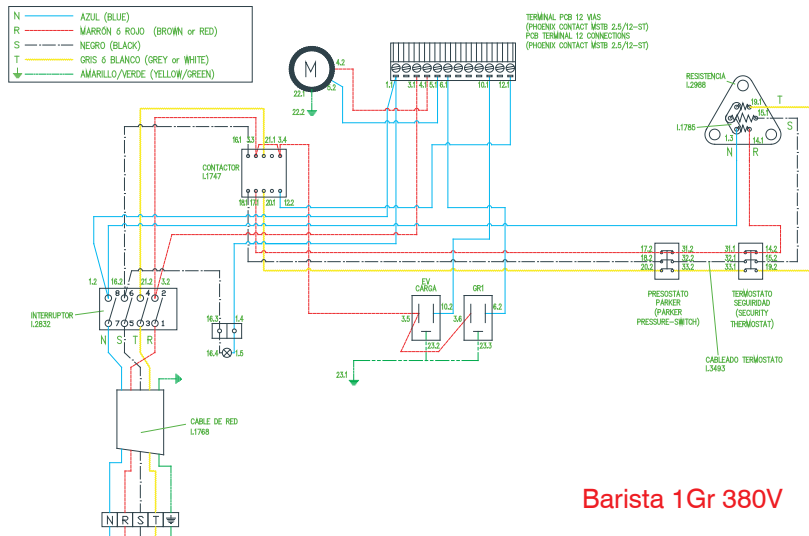
Barista 1Gr 230V
