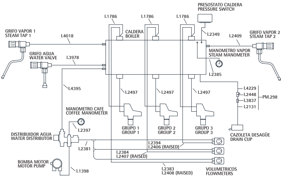
Esquema hidráulico Barista PRO 3GR ■ Barista PRO 3GR hydraulic scheme
